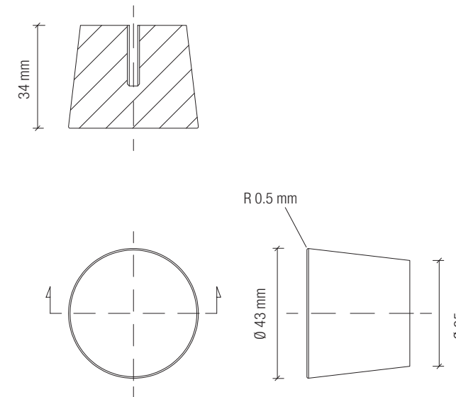
1RV - Maniglia tornita in massello di rovere naturale. 1RV - Handle turned in solid natural oak.
